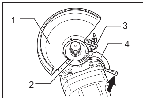
► 1. Protector (guarda) de disco 2. Caja de rodamientos 3. Tornillo 4. Palanca
